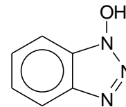
HOBt
