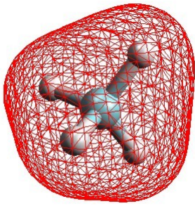
MO \sigma_1
