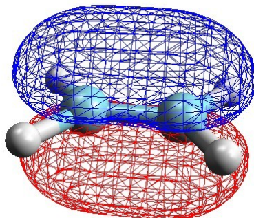
MO \pi \text{ HOMO}
