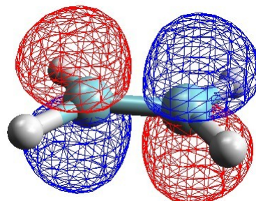
MO \pi^* \text{ LUMO}
