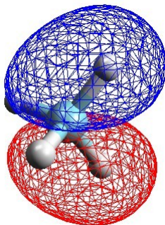
MO \sigma_2
